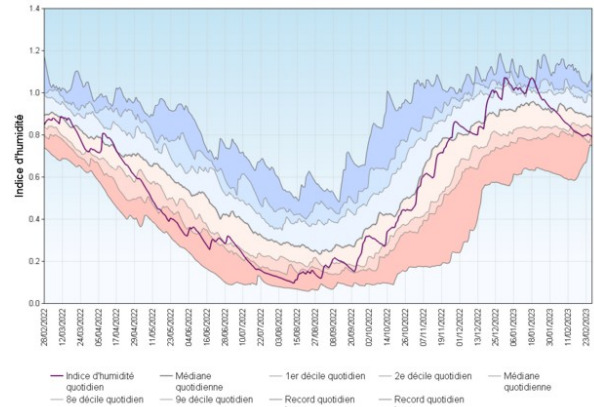
Indice d'humidité des sols agrégé Côtes-d'Armor 28 février 2022 au 27 février 2023
